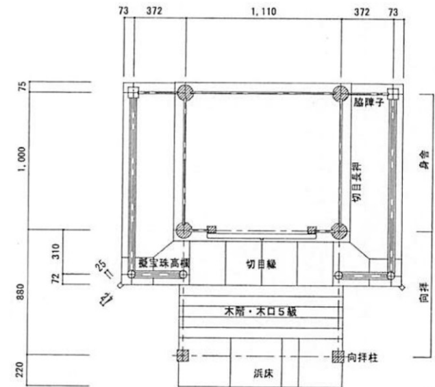
図10 本殿平面図
